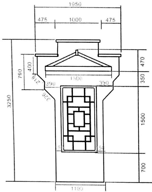
左侧面图
